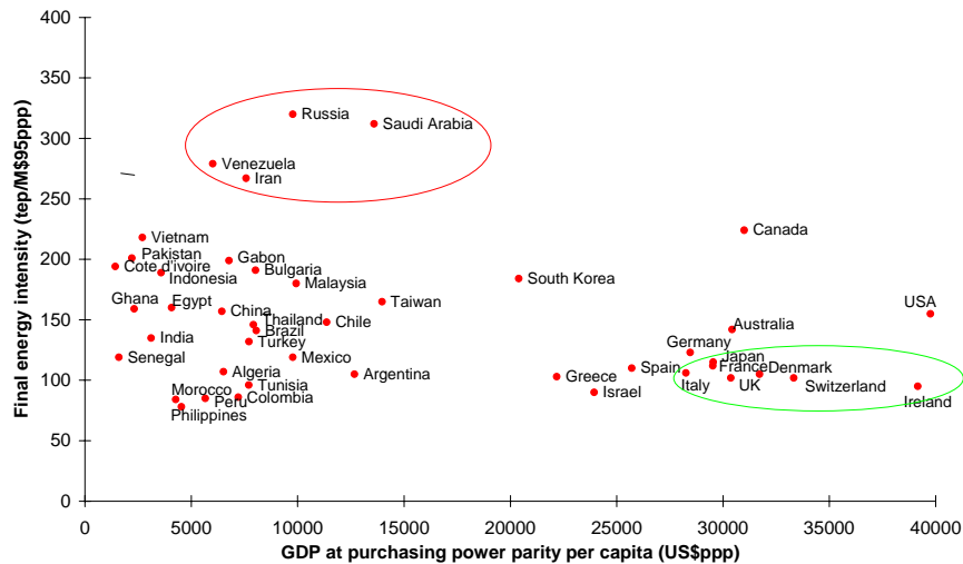
Figure 2.12: Final energy intensity and GDP per capita (2006) Intensité finale et PIB par habitant
